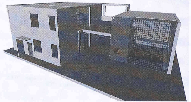
Bild 4. Anwendung des Programms „Soundspace“ auf ein rekonstruiertes Gebäude von Guisepppe Terragni. Beim Durchwandern des dreidimensionalen Modells wird die eigene Stimme in jedem Raum entsprechend der Geometrie und der Materialeigenschaften simuliert. Eric van der Mark
