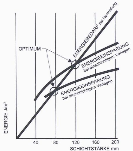
Bild 1. Energetisches Optimum für Mineralwolle, Wohnhaus-Aussenwand, 30% Fenster, Standort Luzern
