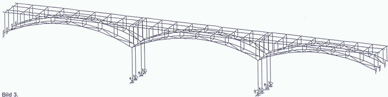
Bild 3. Statisches System
