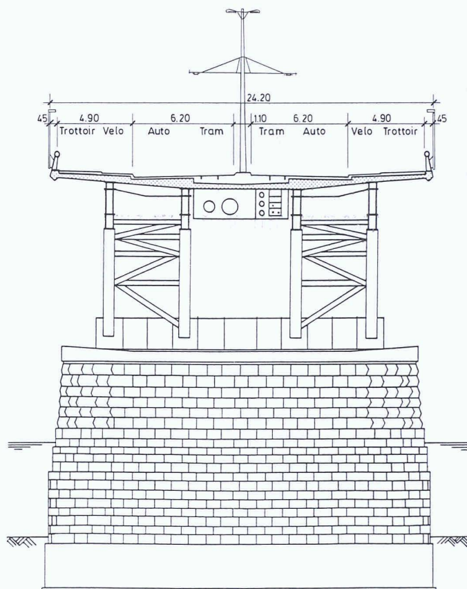
Bild 2. Brückenquerschnitt
