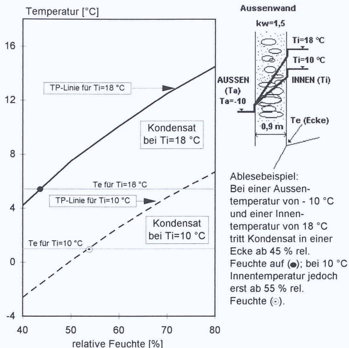
Bild 8. Einfluss der relativen Raumlufffeuchte auf die Taupunkttempera- tur (TP)
