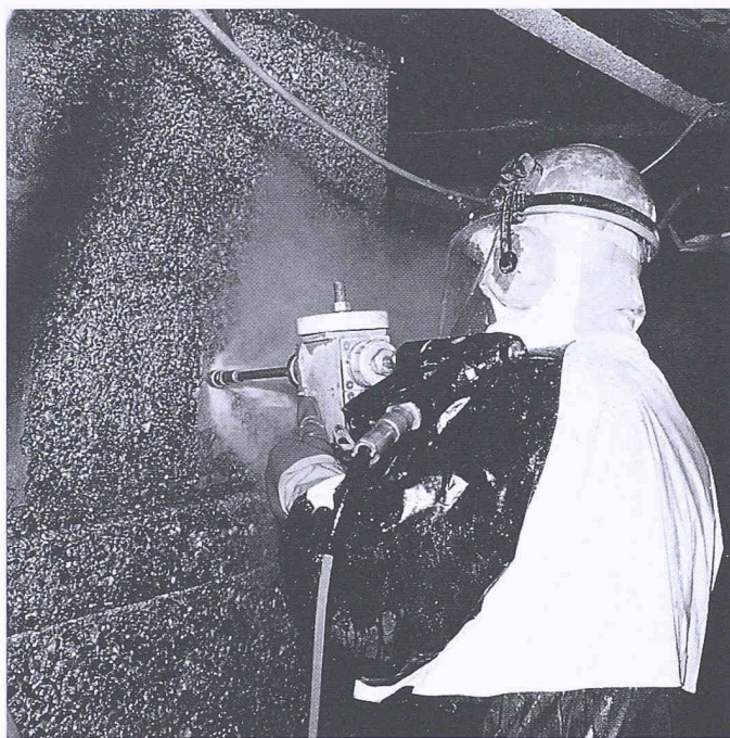
Bild 3. Lanzenführer beim Betonabtrag und Aufrauen des Traggrundes mittels Wasser-Höchstdruck 2000 bar
