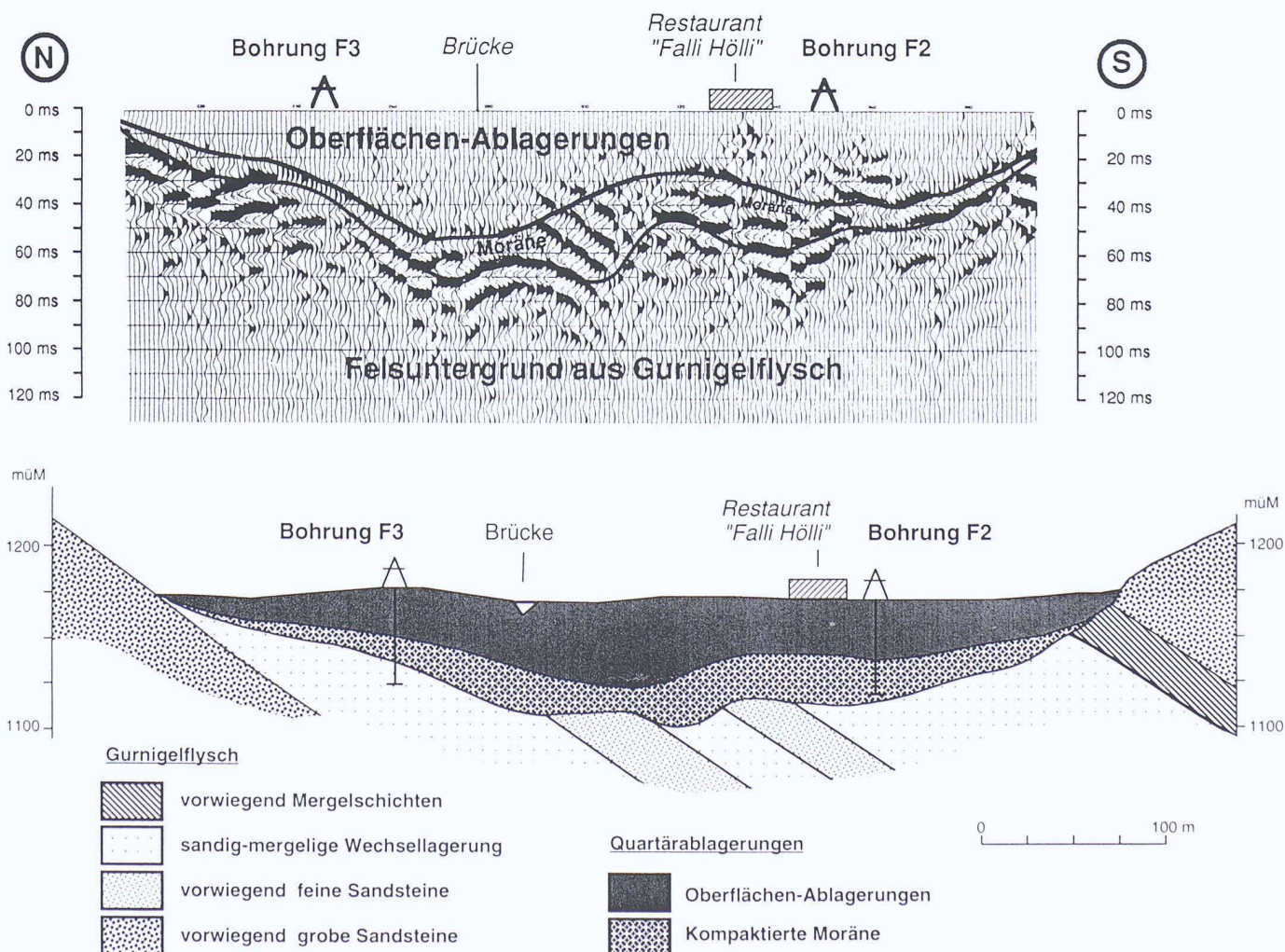
Bild1. Seismisches Profil und Geologische Interpretation
