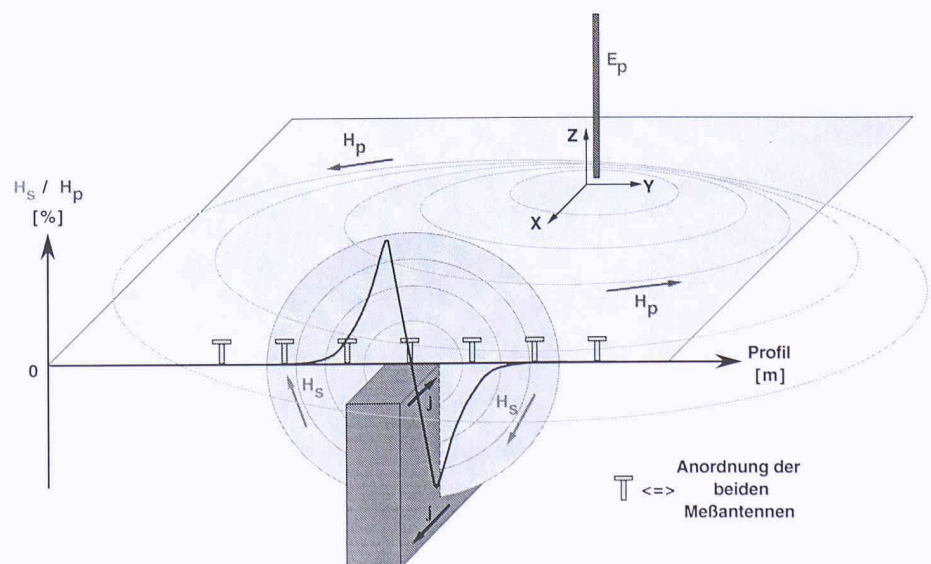
Bild 2. Prinzipische Skizze VLF-EM-Methode
