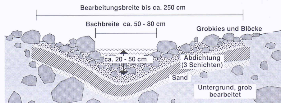
Bild 5. Schnitt durch ein neu angelegtes Fliessgewässer
