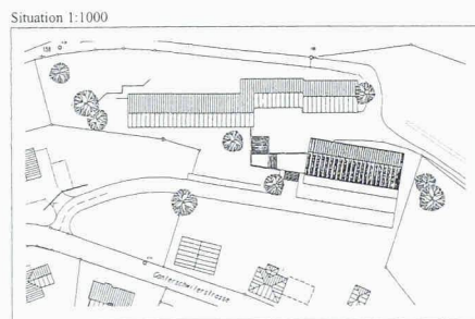
Mehrzweckanlage in Oberhelfenschwil. Projekt von Fredy Kull, Oberhelfenschwil, zusammen mit dem Architekturbüro Walter Boltshauser, Bütschwil. Situation
