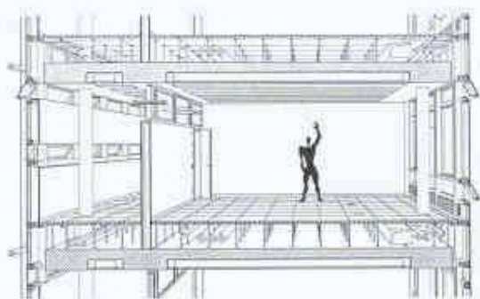
Raummodule Finger, Ost und Nord. Die Raumhöhe (netto) beträgt 2,90 m. Innenraumaufnahmen (Pläne und Bilder: S.A.R., Zürich/Agno)
