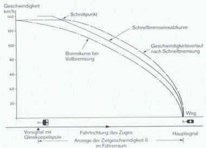
4 Wirkungsweise der Zugsicherung ZUB nach dem Überfahren eines Signals bei Warnung
