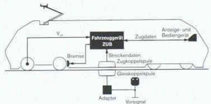
3 Prinzipaufbau der Zugsicherung ZUB
