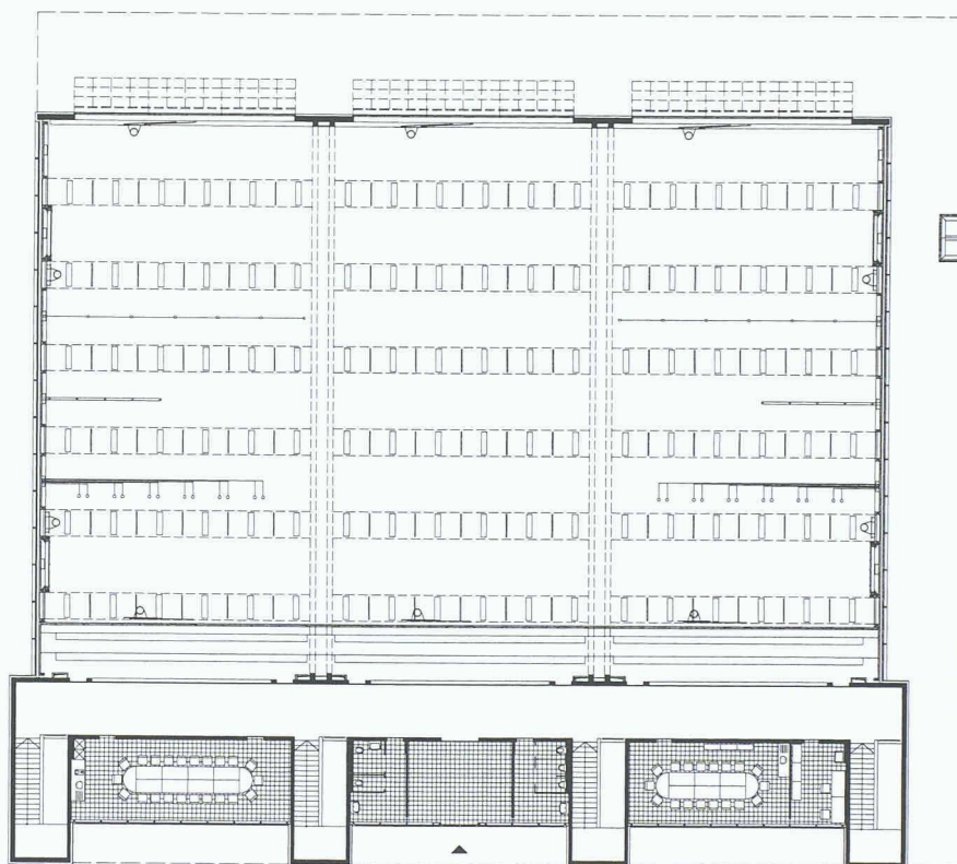
Südfassade (oben). Erdgeschoss (Mitte). Unter- geschoss (unten). Mst. rd. 1:450
