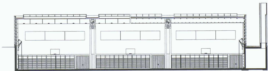
Westfassade (oben). Längsschnitt Halle (Mitte oben). Längsschnitt Vorbau (Mitte unten). Nordfassade (unten). Mst. rd. 1:450
