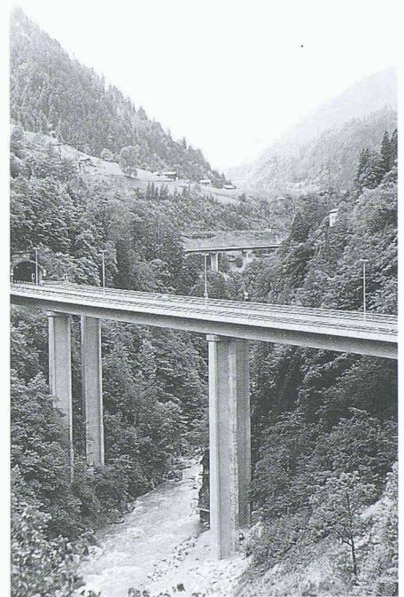
1 Gesamtübersicht Reussbrücke Intschi der A2 im Abschnitt Amsteg–Meitschli. Der Pfeiler Nord (Talspur) befindet sich vorne rechts
