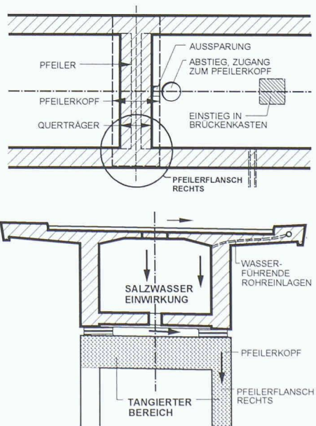
4 Das von der Fahrbahn stammende Salzwasser gelangte durch den undichten Einstieg in den Brückenkasten und von dort an den Pfeiler
