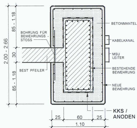
Schematischer Querschnitt des Pfeilerflanschs
