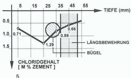
Typisches Chloridprofil, bestimmt an einem Bohrkern aus dem Pfeiler Nord
