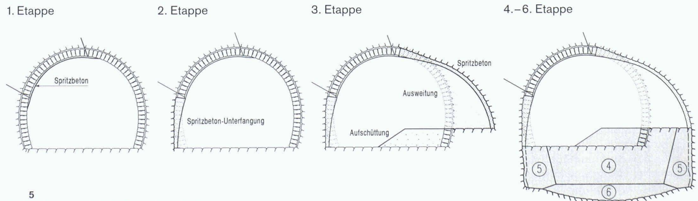
Ausbruchetappen bei der Ausweitung des bestehenden Stadttunnels 1
