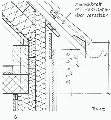
6 Traufe, mit Fusspfette, Betondecke und traufseitiger, keilförmiger Sparrenpfette
