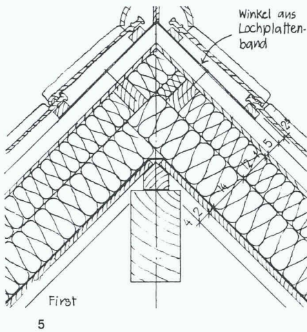
5 First mit mächtiger Firstpfette und den quer zu den Sparren liegenden, schlanken Sparrenpfetten
