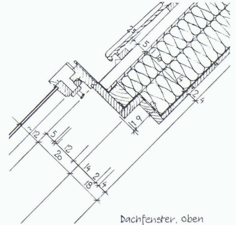
10 Nach wie vor eine Wärmebrücke im Niedrigenergiehaus: Anschlag des Dachfensters an die Dachkonstruktion (Konstruktionszeichnungen: Ueli Schäfer, Binz)
