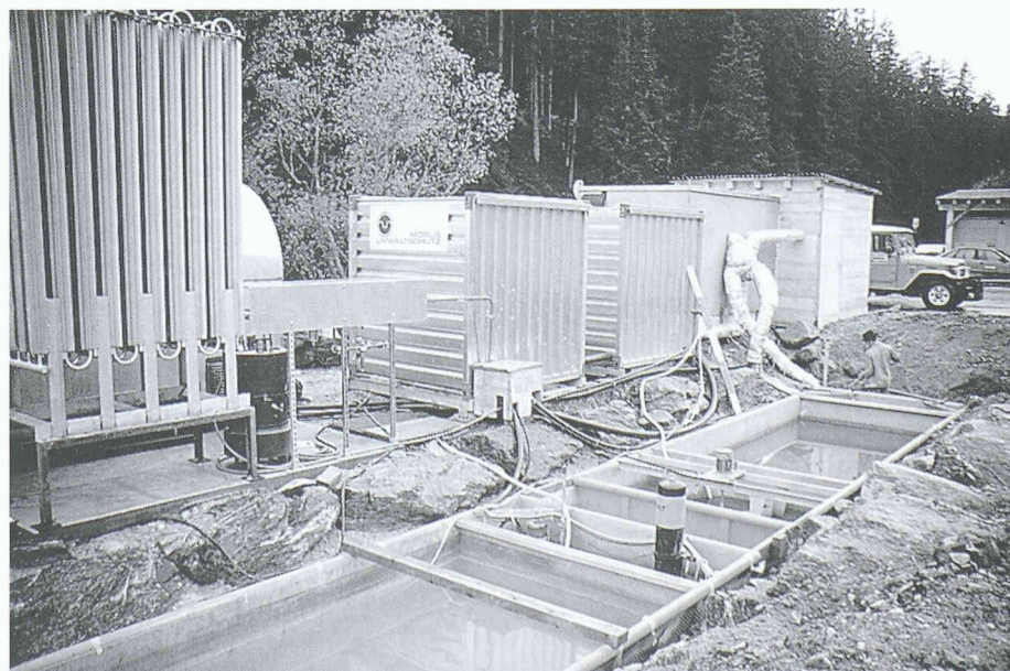
1 Wasseraufbereitungsanlage beim Zwischenangriff Sedrun
