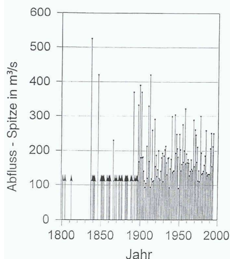
6 Zeitreihe der jährlichen Maximalwerte des Abflusses in der Emme bei Emmenmatt. Die Pfeile deuten historische Hochwasser an, die nicht quantifiziert wurden (nach [5])
