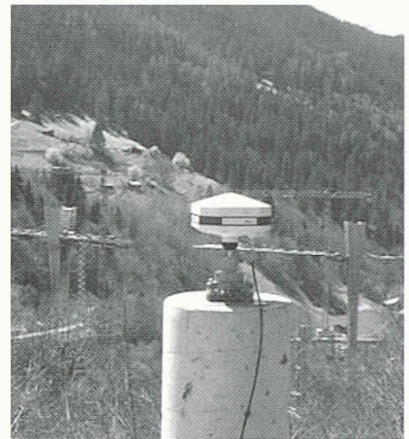
1 GPS-Empfänger im Einsatz für das Grundlagennetz
