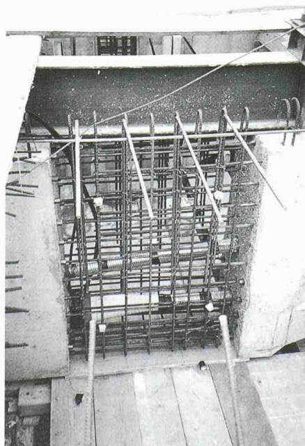
9 Koppelfuge
