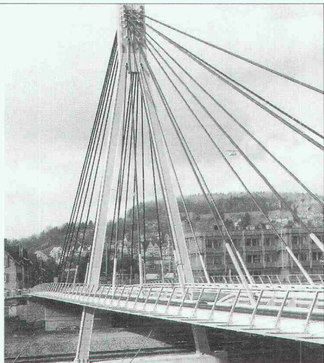
Projekt: Storchbrücke Winterthur Ingenieure: Hölschi + Schurer, Oerlikon
