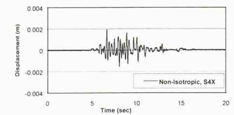
12 Verschiebungsantwort in transversaler Richtung für das taiwanesisches Erdbeben
