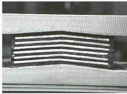
10 Gummilager unter grossen Scherverformungen
