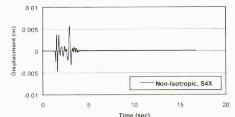
13 Verschiebungsantwort in transversaler Richtung für das Northridge-Erdbeben
