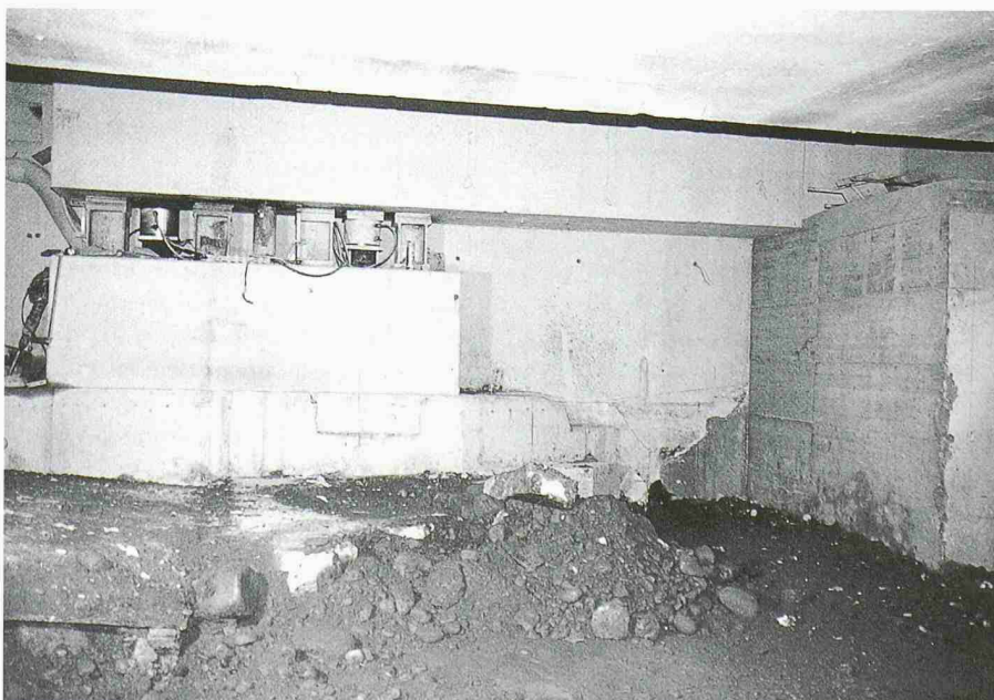
8 Fertiges Tragsystem mit Pfahlbankett, Pressensystem und Träger
