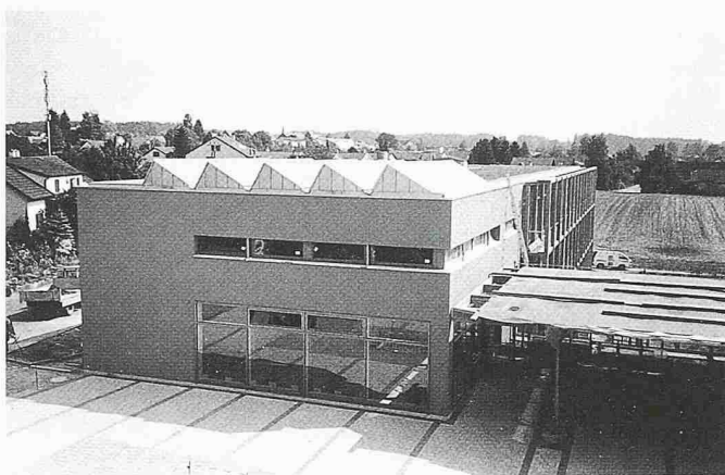
Erweiterungsbau des Oberstufenzentrums Berg TG mit Blech-Sheddach (Vordergrund) und extensiv begrüntem Foamglas-Gefälledach
