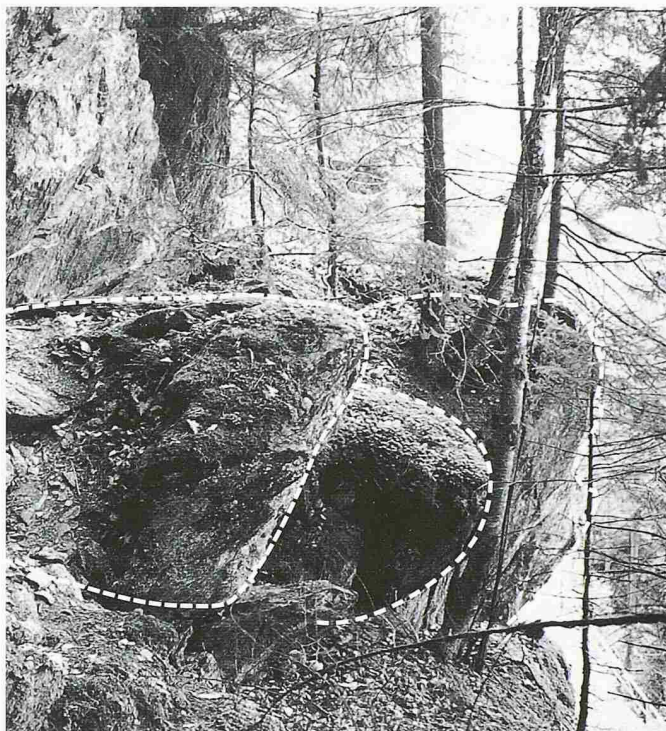
8 Drei klar erkennbare «labile Blöcke» im Teil 2a (V 0,5 bis 4 m 3 )
