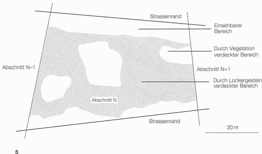
Schematische Darstellung der einsehbaren und verdeckten Bereiche im Abschnitt N ober- und unterhalb der Bristenstrasse
