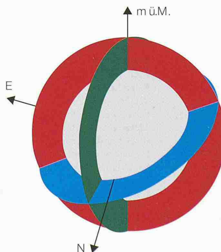
9 Anschauliche Darstellung der Trennflächenebenen in einer Kugel (grau = Fels) mit Schieferung (rot) und zwei Trennflächenscharen (grün, blau)
