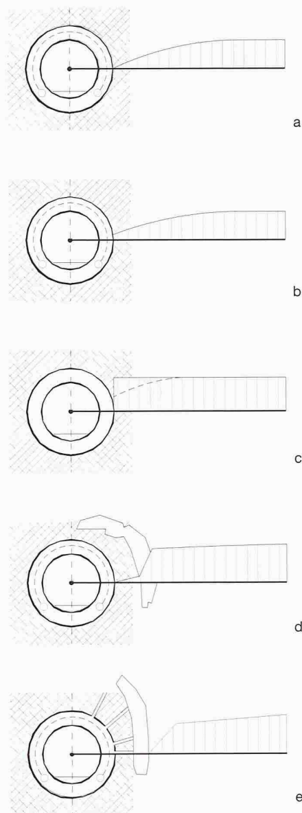
Wasserdruckaufbau beim Zufluss zum Tunnelhohlraum. a: drainierter Tunnel, b: Teilentspannung des Wasserdrucks, c: wasserdruckhalten der Tunnel, d: Wasserverdrängung durch Injektionen, e: zusätzliche Druckentlastung durch Entwässerungsbohrungen
