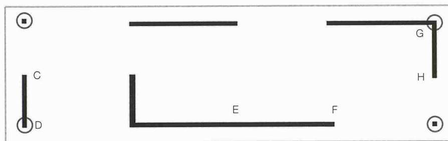
Grundriss 1. Geschoss
