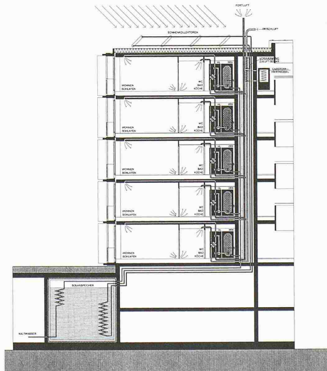
Haustechnikkonzept Wohnanlage Wohnen am Lohbach, Innsbruck (Bild: Architekturbüro Baumschlager & Eberle ZT GesmbH)
