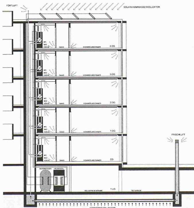
Haustechnikkonzept Wohnanlage Mitterweg, Innsbruck (Bild: Architekturbüro Baumschlager & Eberle ZT GesmbH)
