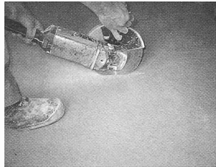
2 Einschlitzten des Traggrunds mit der Fräse
