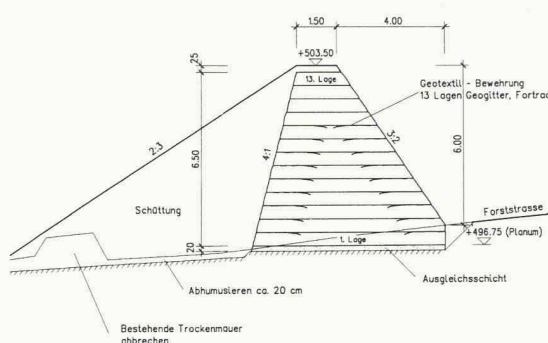
5 Schnitt Leitdamm
