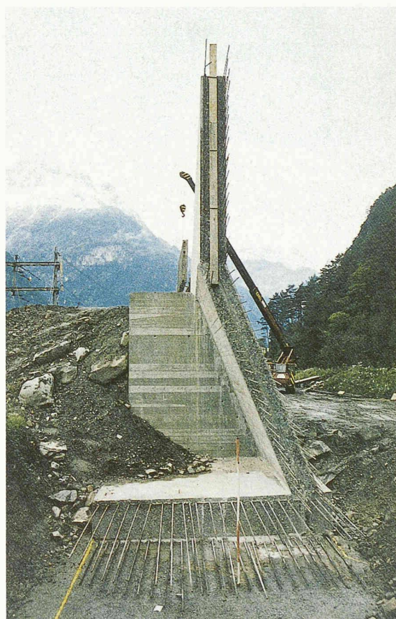
6 Seitenansicht Auffangmauer
