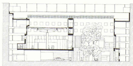
Querschnitt durch den Hof und Längsschnitt
