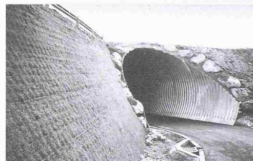
Geh- und Radwegunterführung Staatsstrasse Nr. 13 Wil-Wattwil
