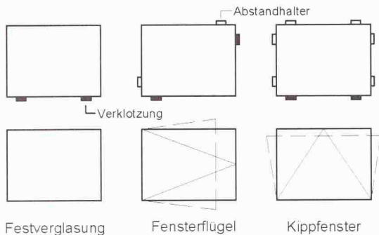
6 Verklotzungsarten
