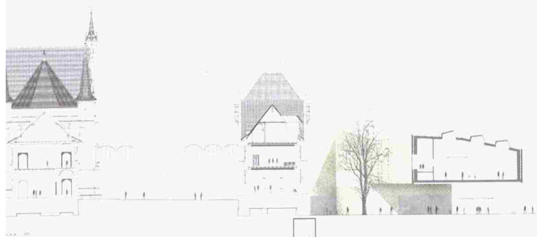
Erweiterung Schweizerisches Landesmuseum in Zürich: Siegerprojekt von Christ und Gantenbein aus Basel. Obergeschoss und Erdgeschoss (links oben), Schnitte (unten) und Situation zwischen Hauptbahnhof und Platzspitz (oben) (Bilder: Christ und Gantenbein)
