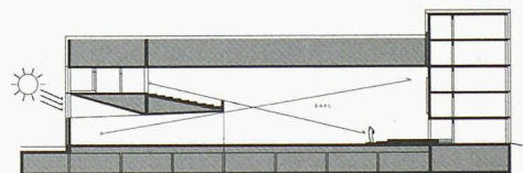
Querschnitt durch den Hallenteil und den Kopfbau
