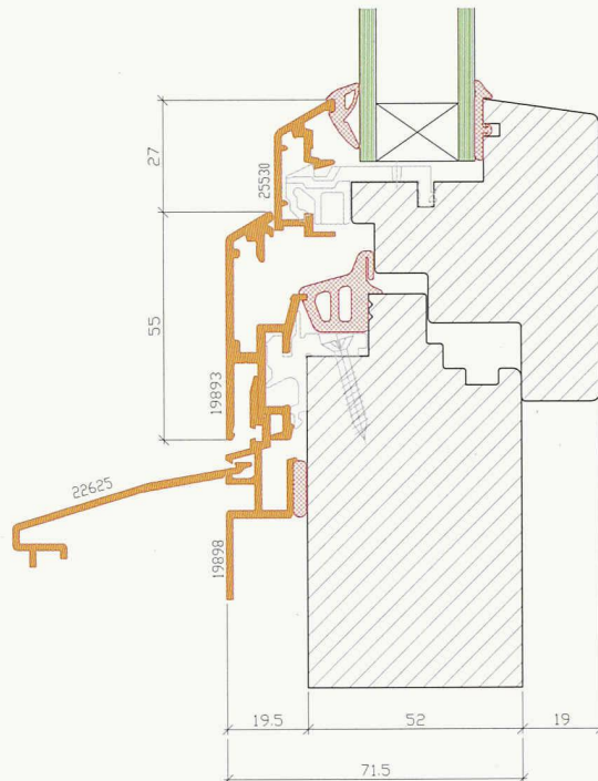
Konventionelles Holz-Metall-Fenster. Die Ansichtsbreite des Flügelrahmens beträgt 72 mm. Massstab 1:2 (Bild: WFT)
