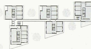
Grundriss 1. Obergeschoss der Baufelder 8 und 9. Eine einfache Wohnungstypologie der Etagenwohnungen (1. Rang, Regina + Alain Gonthier)
