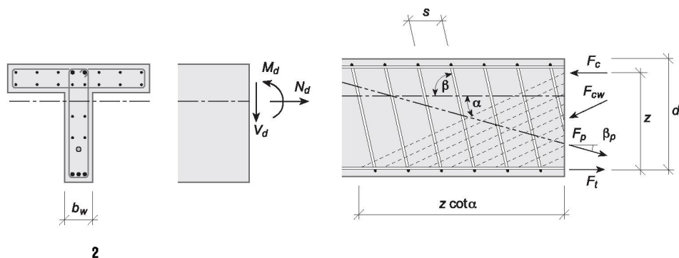
Spannungsfeld für die Bemessung von Trägerstegen
