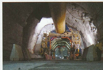
Am zweiten Tagungstag finden Exkursionen auf die Baustellen des Gotthard-Basistunnels in Bodio, Faido, Sedrun und Amsteg statt. Oben: Tunnelleinsicht Faido (Bild: FGU)
