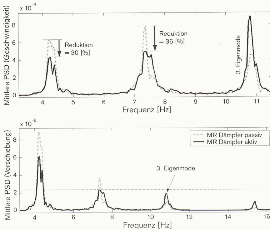
Experimentelle Ergebnisse: Vergleich zwischen adaptiver und passiver Dämpfung (Bilder: Empa Dübendorf)
