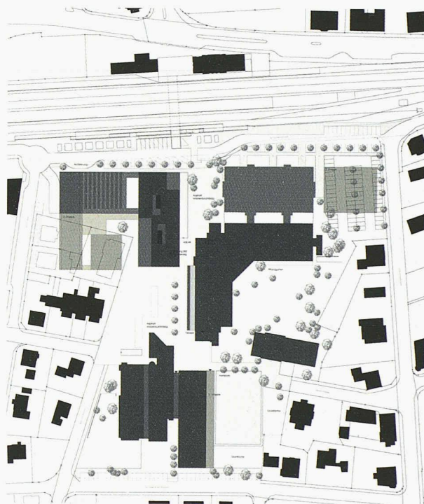
Der winkelförmige Neubau mit den möglichen Erweiterungen (zur Ausführung empfohlen, Antoniol + Huber + Partner)
