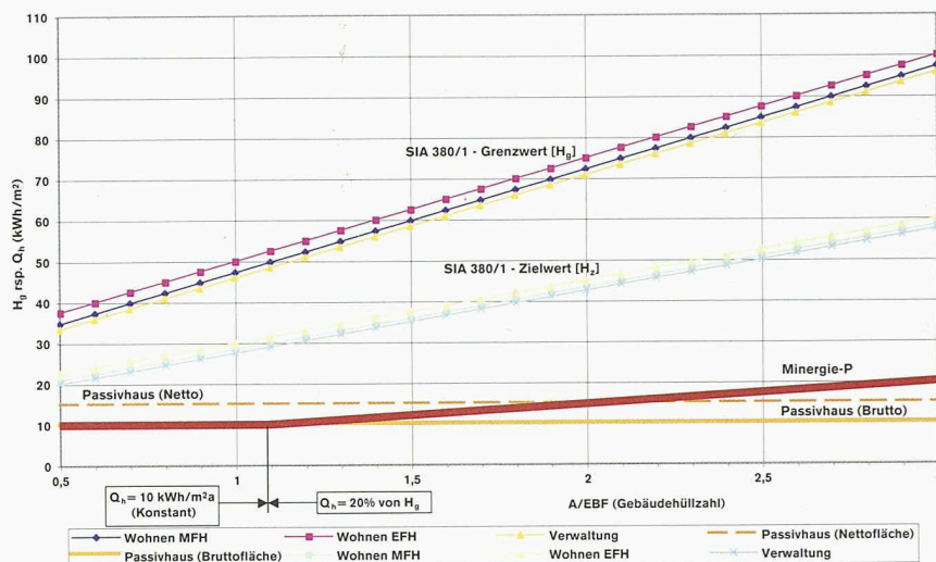
Vergleich SIA 380/1 mit Minergie (Vorschlag der Q_n -Definition)
