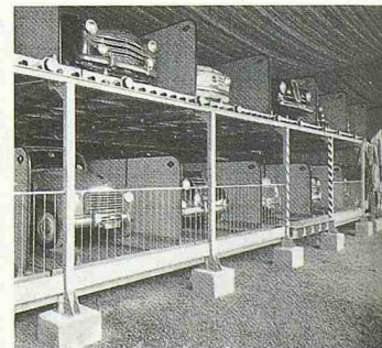
Bild 3. Untere und obere Boxenreihe sowie Mittelteil-Traggerüst mit Wagenentnahmepunkte (Schleibühne fehlt)
