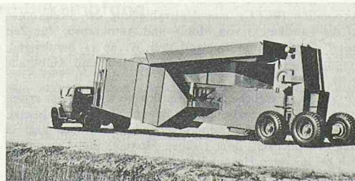
Bild 1. Der zweiteilige Mischturm mit eingebauten Fahrwerken kann paketweise auf Sattelschleppern zum Mischplatz gefahren werden
