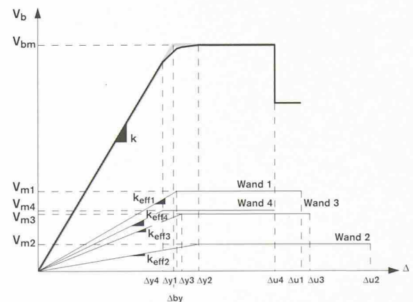
Kapazitätskurve des fiktiven Beispielgebäudes
