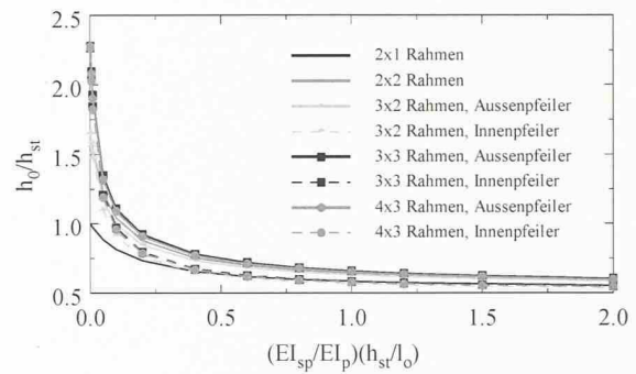
Verlauf der Höhe des Momentennullpunktes h_0 (bezogen auf die Stockwerkshöhe h_{st} ) in Funktion der relativen Steifigkeit der Riegel zur Steifigkeit der Pfeiler
