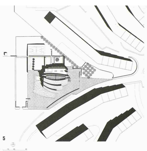
5 Die Situation der Kirche auf einem dreieckigen Gelände im Quartier Tor Tre Teste (Mst. 1:3000)
