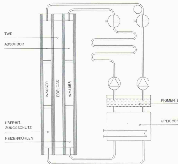
Flüssigkeitsdurchströmte Glasfassade, Schema
