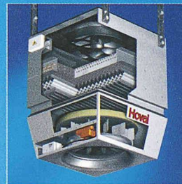
TopVent® DKV.
