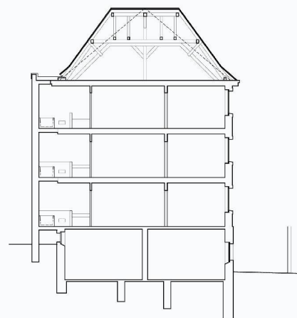
Areal 1, 1. Rang: Querschnitt mit Erweiterung
