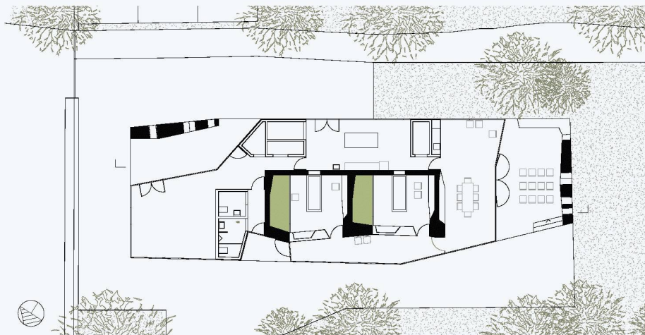
03 Grundriss
