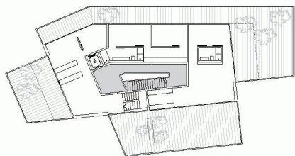
03 Dachgeschoss, Mst. 1:700
