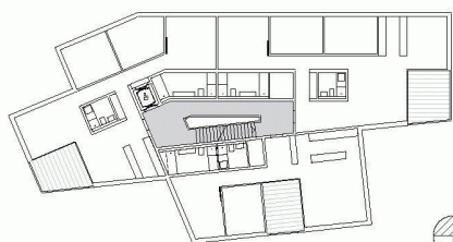
05 Erdgeschoss, Mst. 1:700
