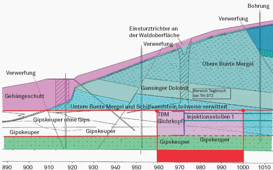
04 Geologisches Längenprofil im Bereich des Tagbruchs bzw. des instandzusetzenden Abschnitts
